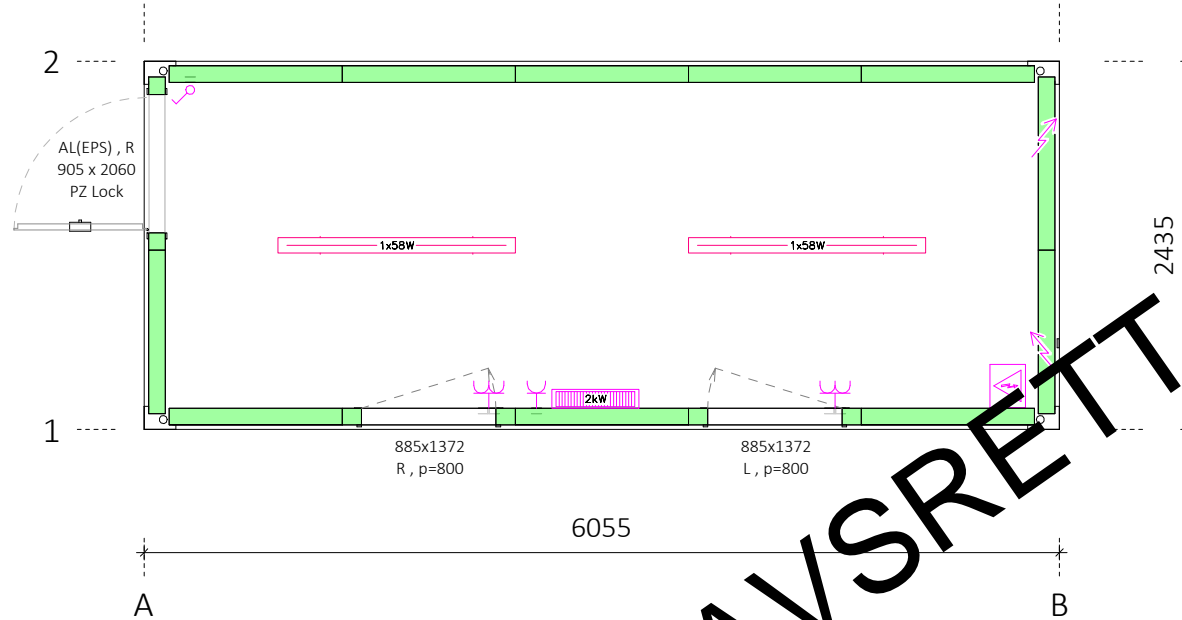
Floor Plan 1 : 50
